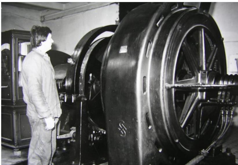
Stav těžního stroje v roce 2000, archiv Hornického skanzenu Mayrau
